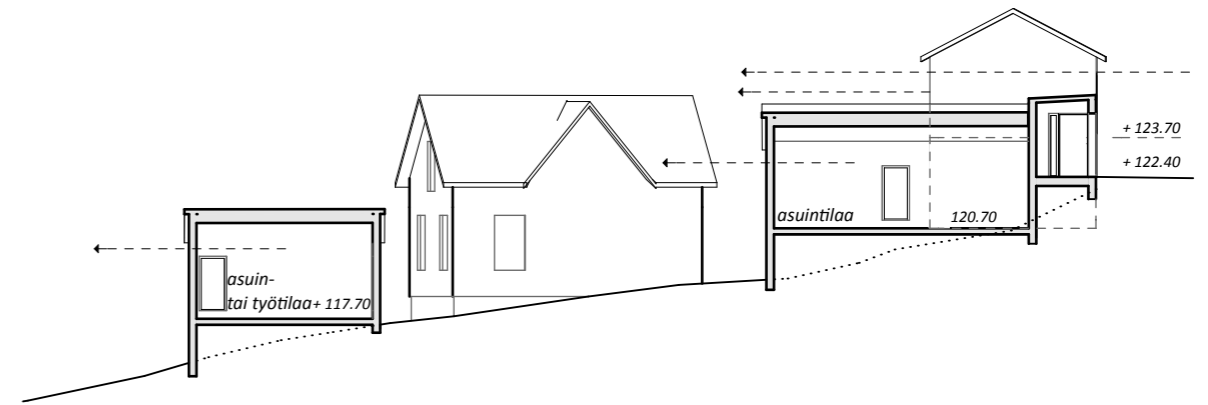
Leikkaus T10A 1:250
