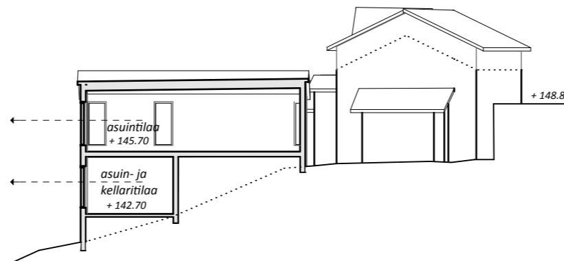
Leikkaus T1Au 1:250
