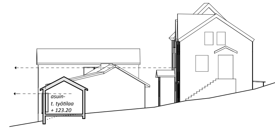
Leikkaus T9A 1:250
