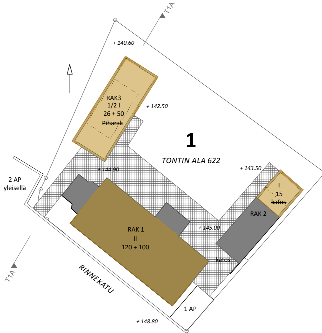
Asemapiirros 1:250
