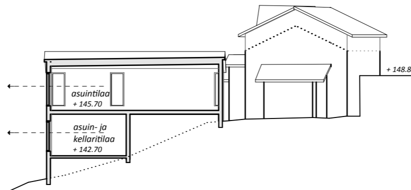
Leikkaus T1A 1:250
