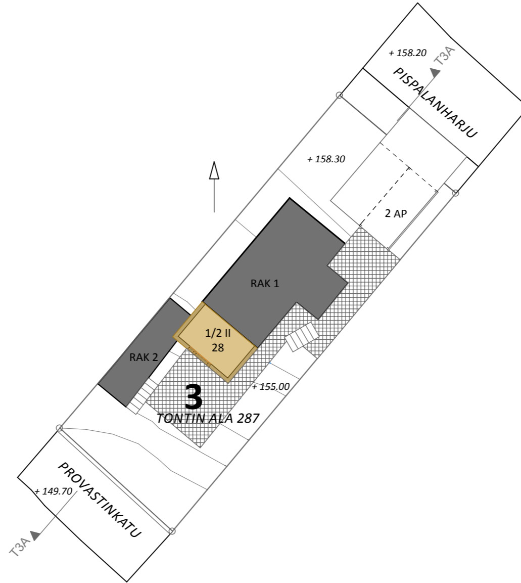
Asemapiirros 1:250
