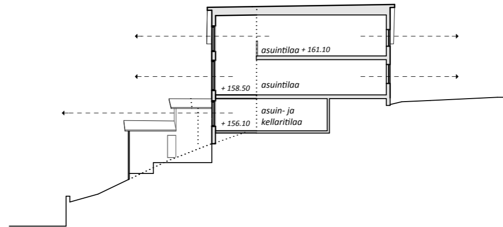
Leikkaus T3A 1:250
