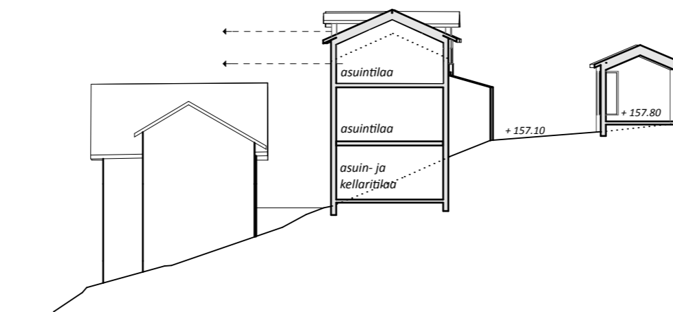
Leikkaus T2Au 1:250
